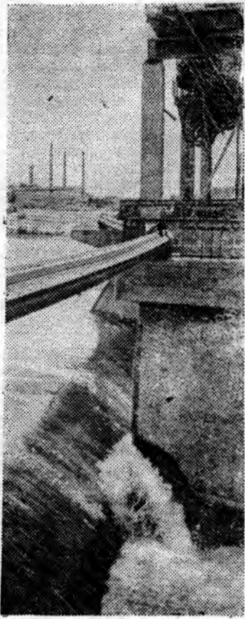
КРАСНОЯРСКИЙ край. На Назаровской ГРЭС идет строительство и монтаж блока, где будет установлен уникальный генератор мощностью 500 тысяч киловатт. НА СНИМКЕ: вид на ГРЭС через водосливную плотину. Фото Ю. Бармина. Фотохроника ТАСС.
